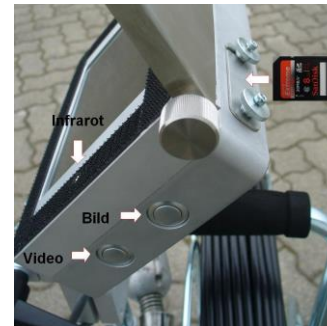
Integrierter SD-Card-Recorder
